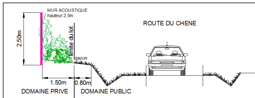
COUPE DE PRINCIPE SUR MUR ACOUSTIQUE
